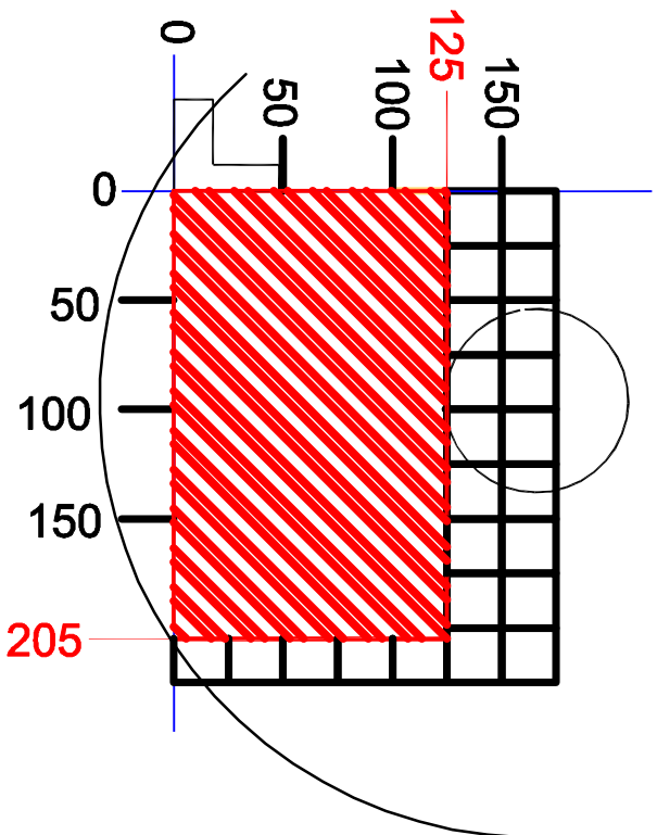
90° : 205 x 125 mm
