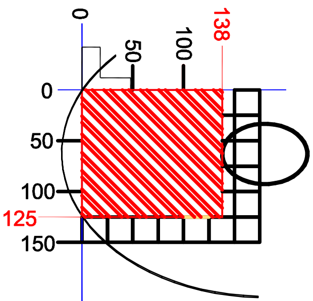
45° : 125 x 138 mm
