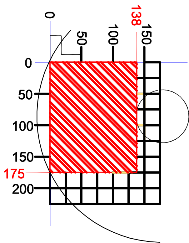
90° : 175 x 138 mm
